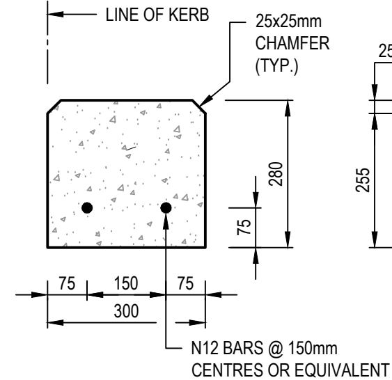
EDGE STRIP (INDUSTRIAL) ④
